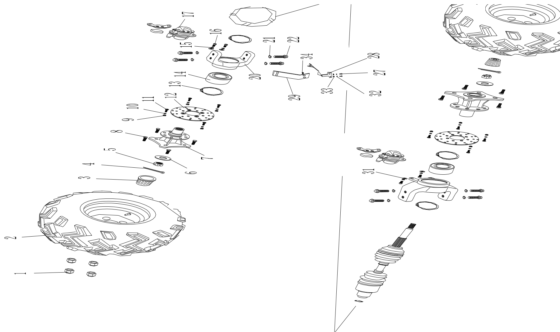
F-5 后传动系统---REAR SHAFT TRANSMISSION.
